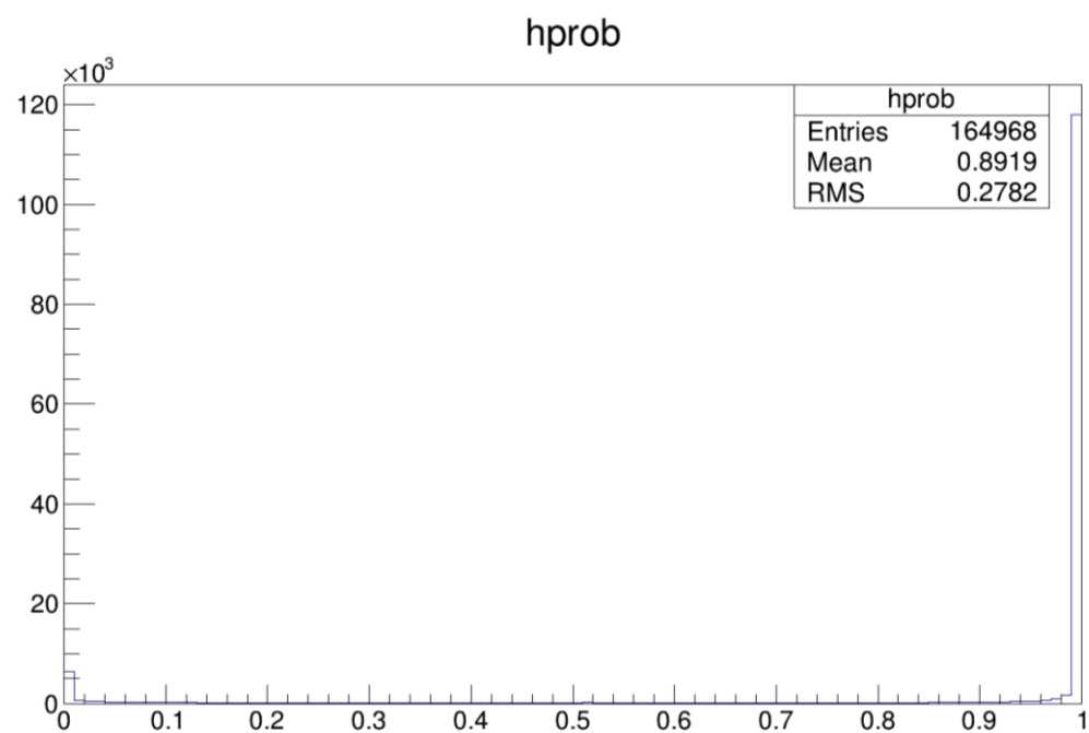
信号蒙卡的PID选择条件
