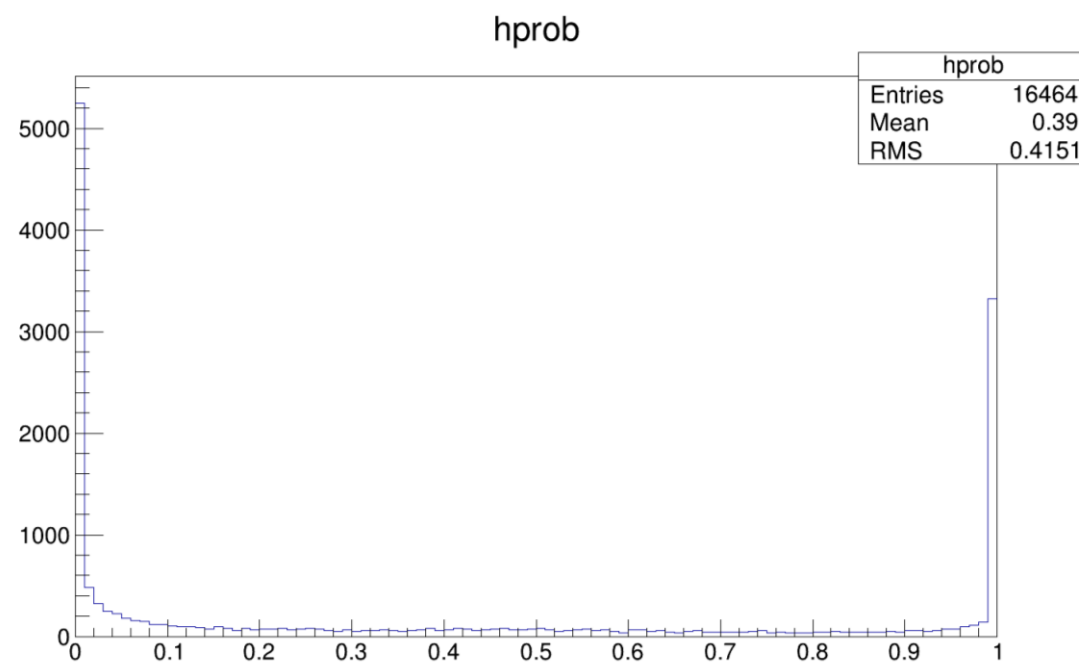
本底蒙卡的PID选择条件
